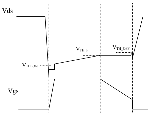
图 1 SP6551FL 的典型波形
